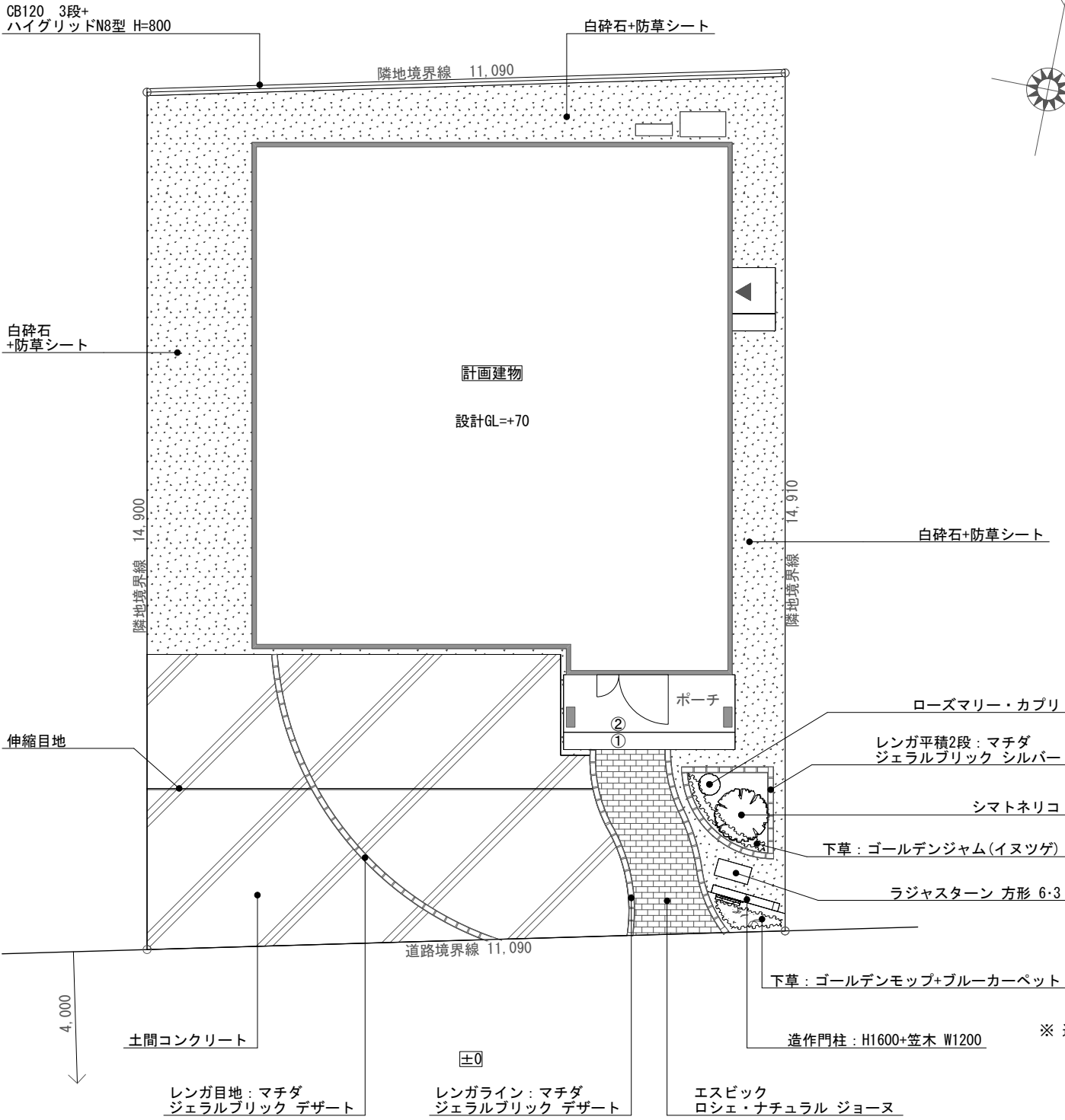
平面図
